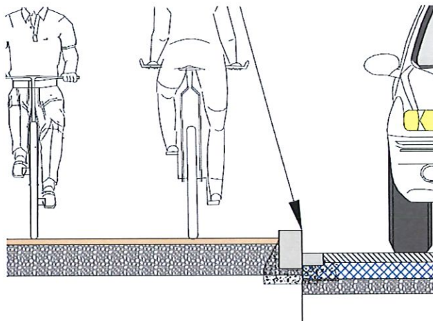
Zoom de détail de la double vue sur la bordure
