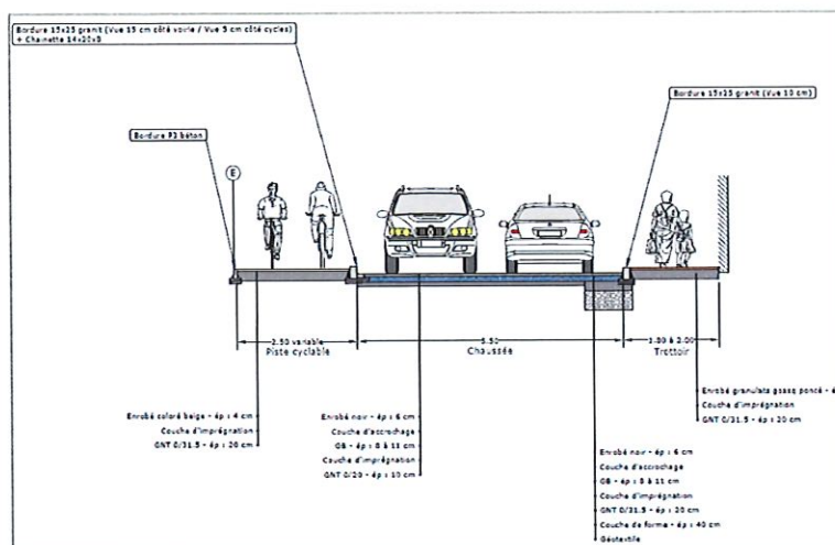
Profil en travers le long du boulevard
